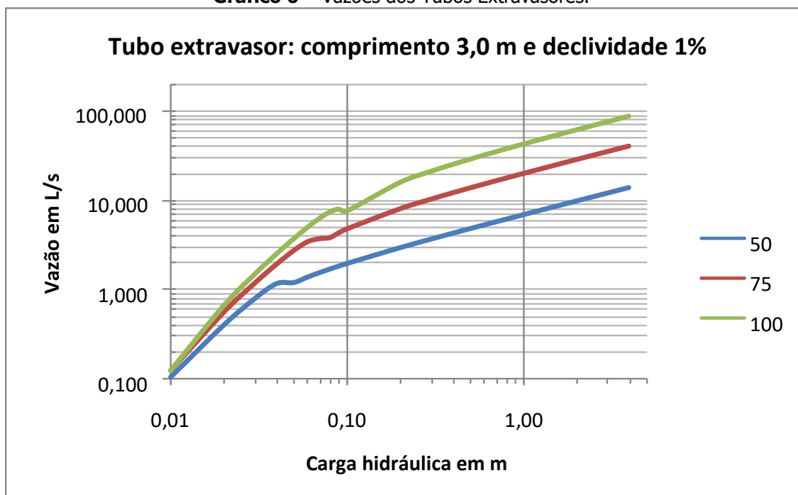
Gráfico 6 – Vazões dos Tubos Extravasores.
