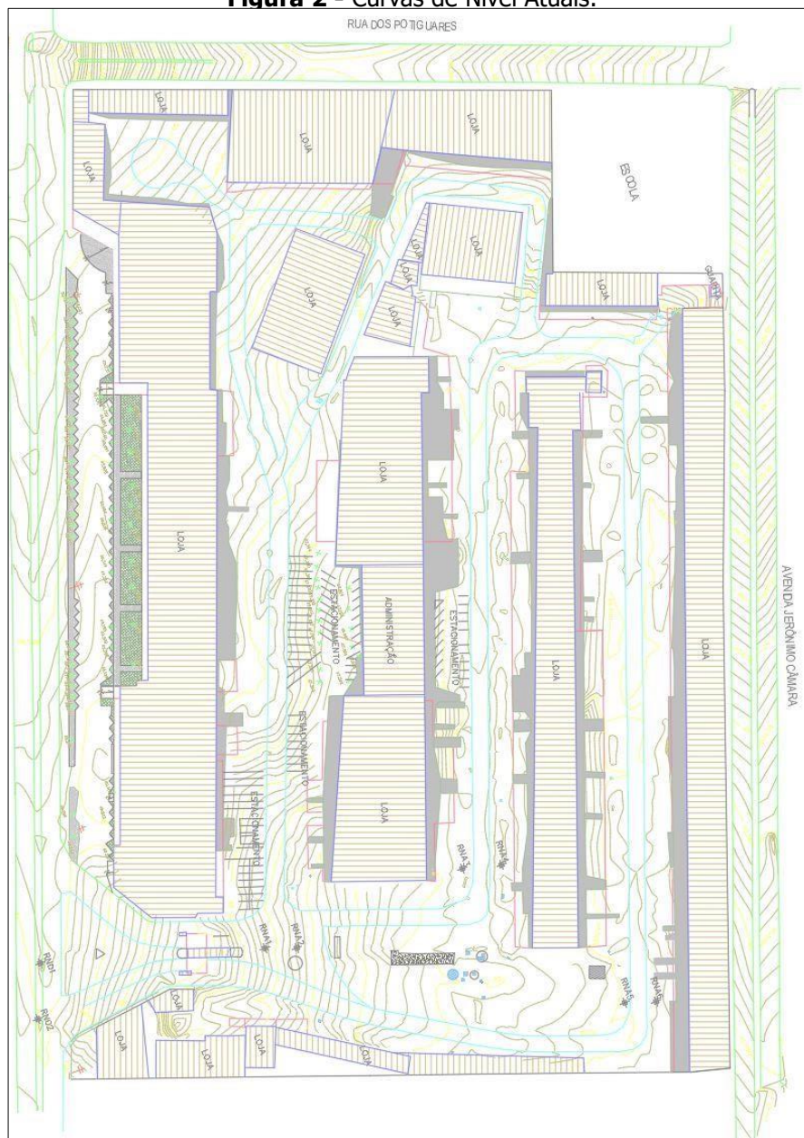
Figura 2 - Curvas de Nível Atuais.
