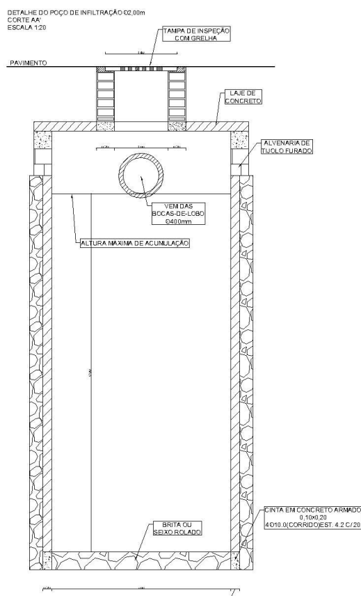
Figura 5 - Corte AA do Sumidouro Adotado como Padrão.
