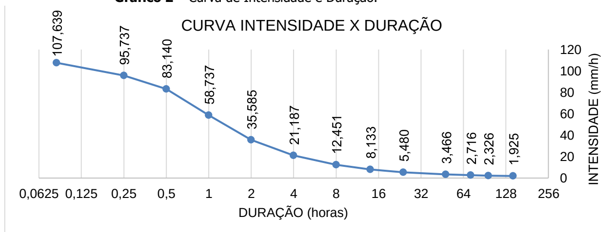
Gráfico 2 – Curva de Intensidade e Duração.
